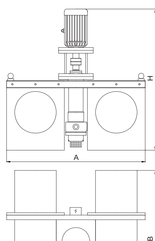
配两只浮桶的泵外形图
