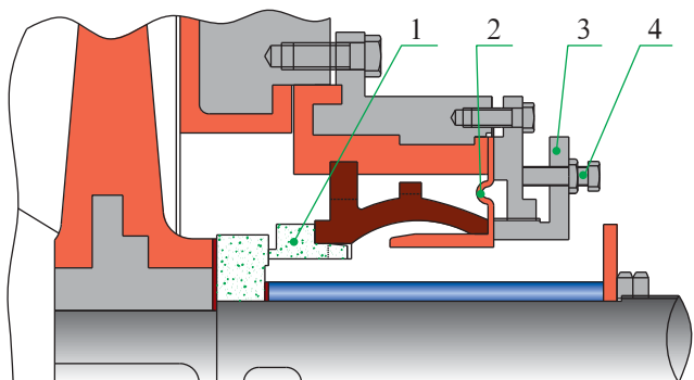
1. 静环 2. 弹性密封环 3. 密封比压调正环 4. 定位螺栓
