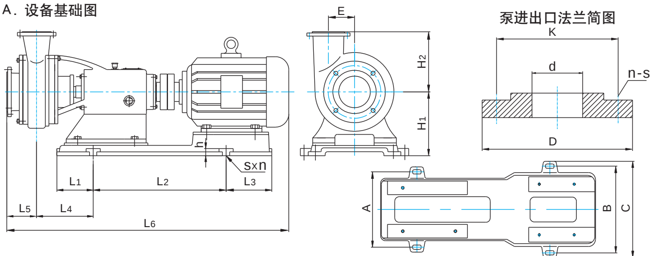
A. 设备基础图
